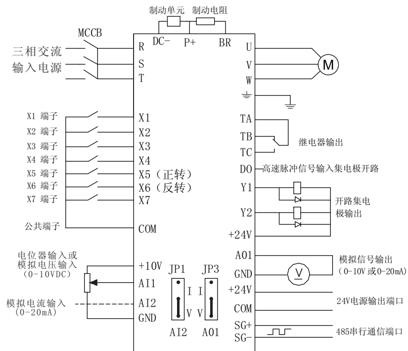
图3-4 基本配线图
