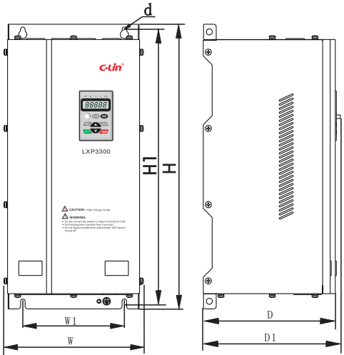
图9-2 (机型B) 变频器尺寸示 图
