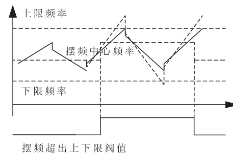
图F6-5 摆频幅度限制示意图
