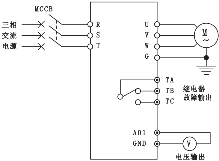
图7-2 范例1接线图
