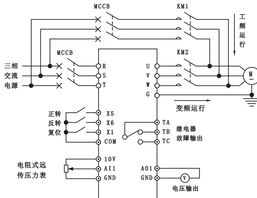
图7-7 范例5接线图
