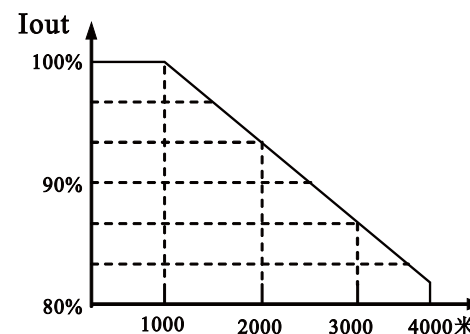
图7-1 变频器降额曲线图
