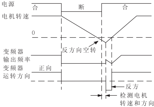
图F2-1转速跟踪起动示意图
