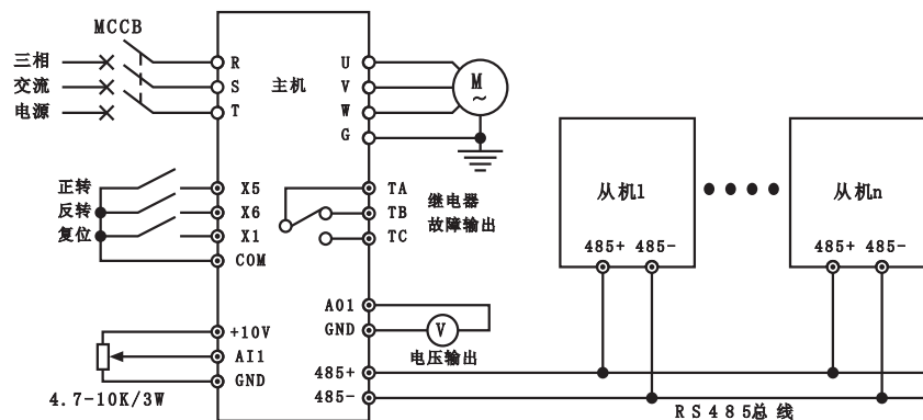
图7-6 范例4接线图
