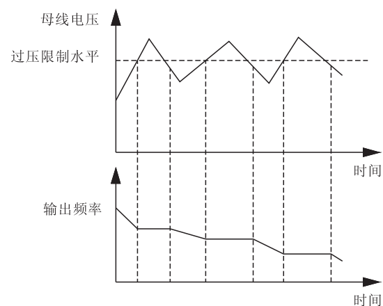
图FA-1 过压限制水平说明示意图
