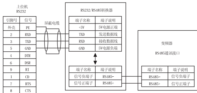
图 3-15 上位机与变频器接口接线图
