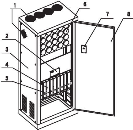
图 2-5 机型C外观图
