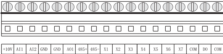
图3-11 控制电路端子1
