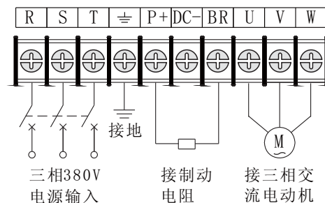
图3-7 主电路端子图2
