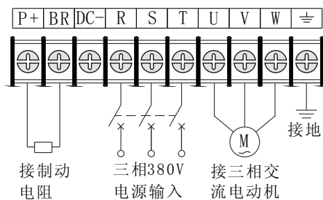
图3-8 主电路端子图3
