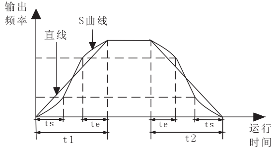
图F2-4 直线与S曲线加减速示 图
