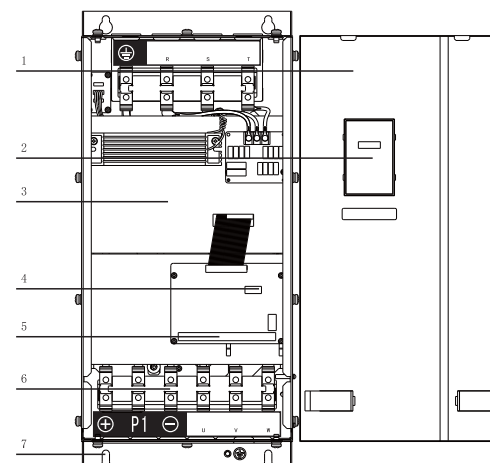
图 2-3 机型B外观图
