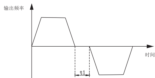
图F2-8 正反转死区时间示 图
