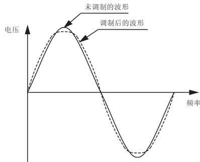
图F5-2 过调制功能示意图
