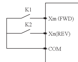
图F6-1 二线式控制模式1示意图
