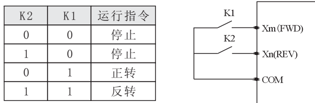
图F6-2 二线式控制模式2示意图
