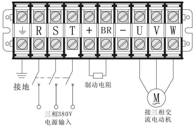
图3-9 主电路端子图4
