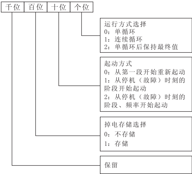
图F9-1 简易PLC运行示意图
