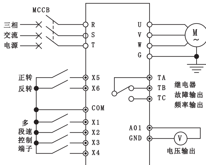
图7-4 范例3接线图
