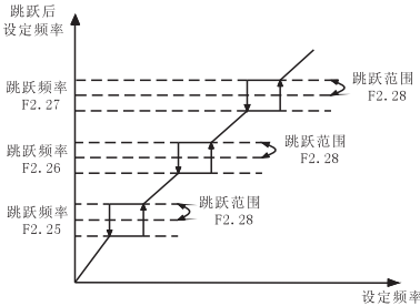
图F2-7 跳跃频率示意图
