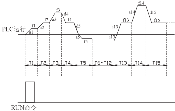
图F9-4 简易PLC运行示图
