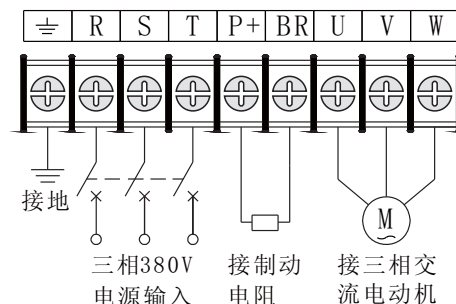
图3-6 主电路端子图1
