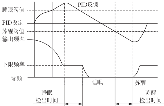
图F8-6 睡眠与苏醒功能示意图
