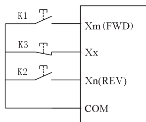
图F6-3 三线式控制模式1示意图
