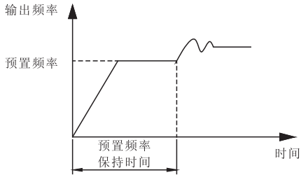
图F8-5 闭环预置频率运行示意图
