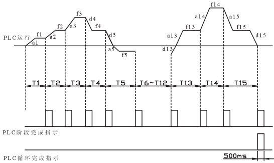
图F9-1 简易PLC运行示意图
