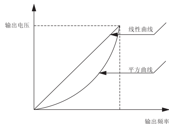
图F3-1 V/F曲线示 图
