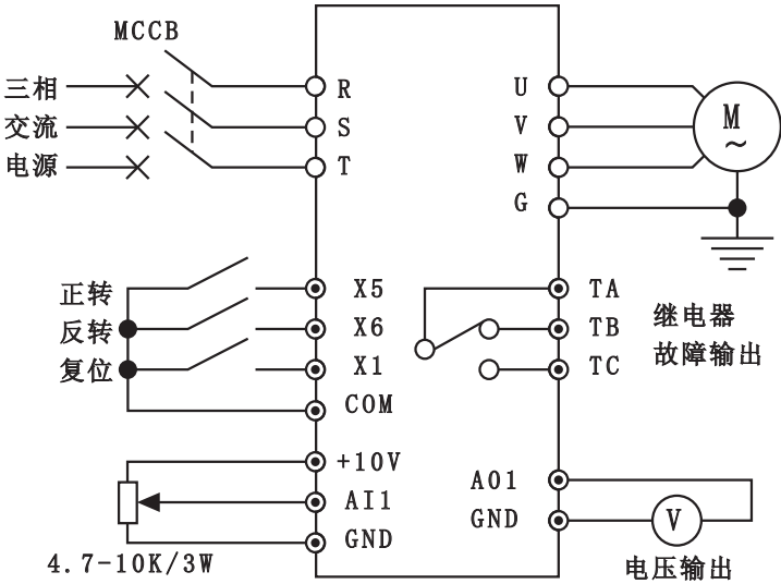
图7-3 范例2接线图
