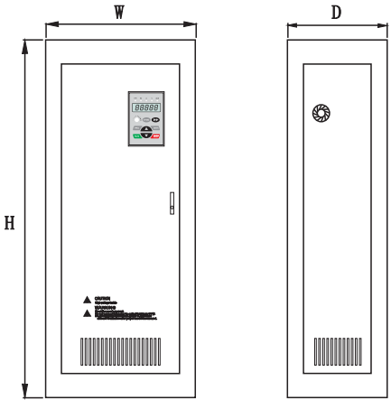
图9-3 (机型C) 变频器尺寸示意图
