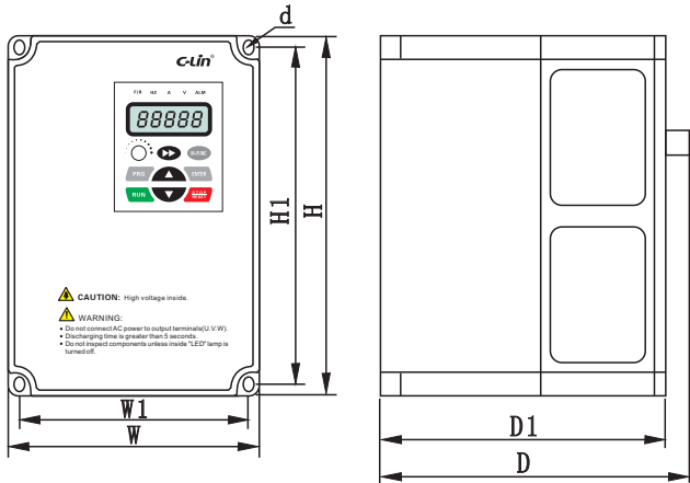
图9-1 (机型A) 变频器尺寸示意图
