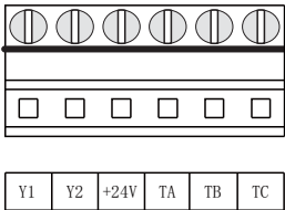
图3-12 控制电路端子2
