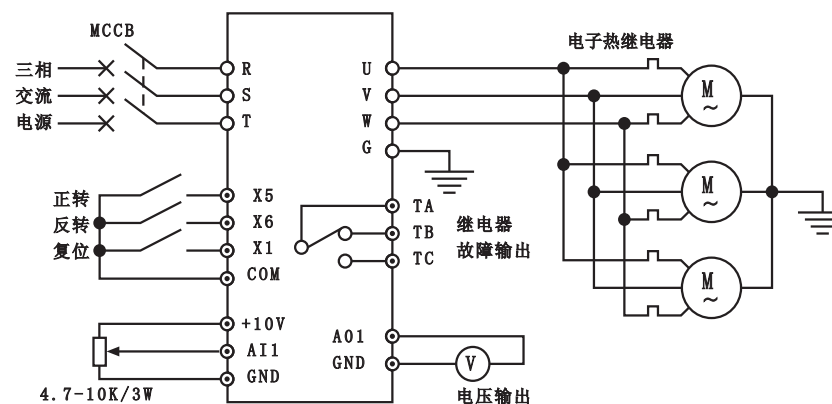
图7-5 范例4接线图
