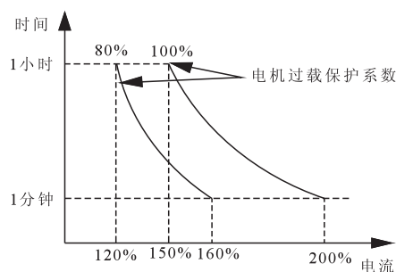
图FA-5 电机过载保护系数设定示意图
