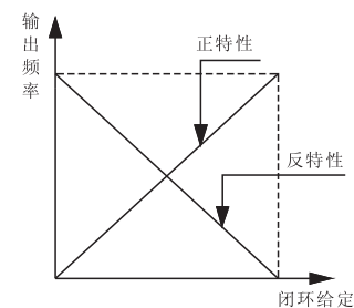
图F8-3 正负特性示意图
