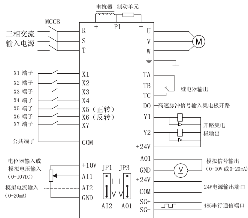
图3-5 基本配线图
