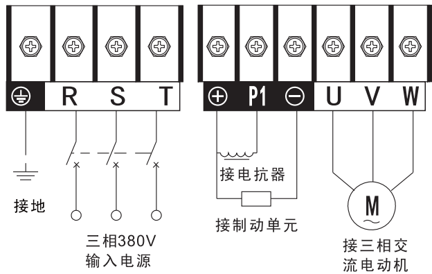
图3-10 主电路端子图5
